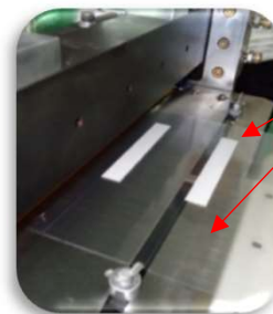
連続短冊加工・移載部
