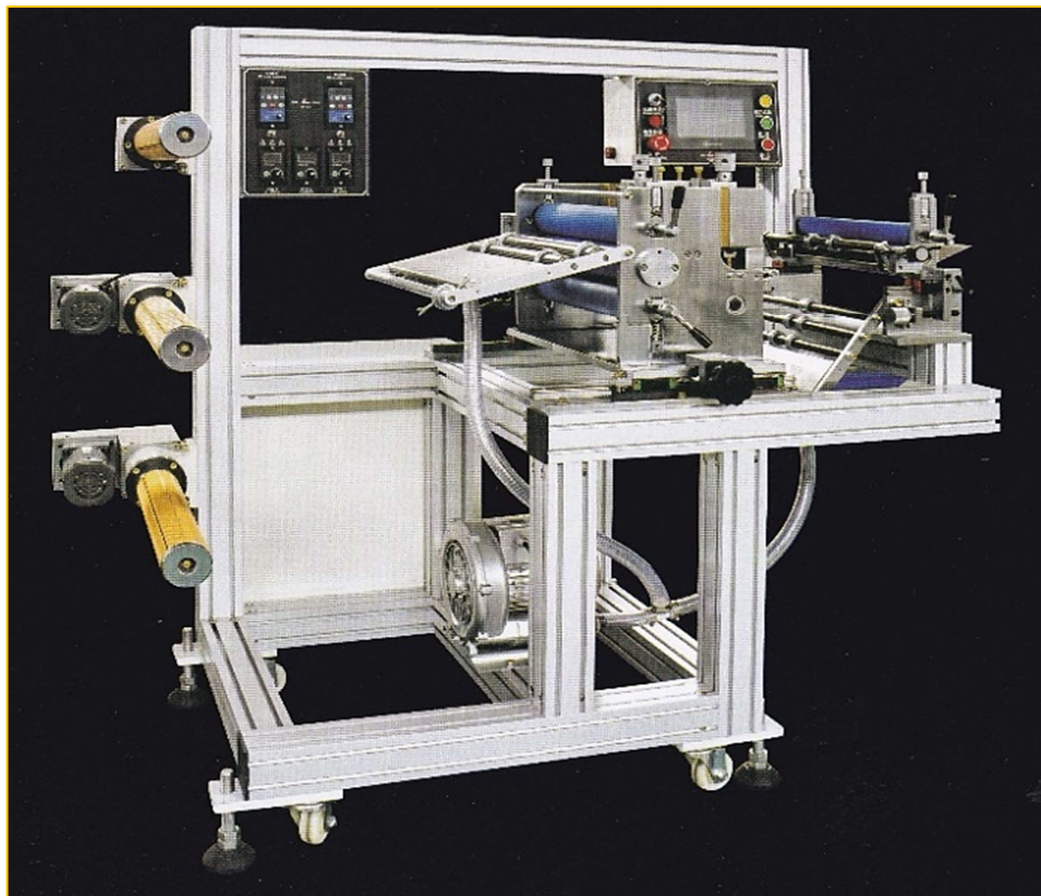
基材供給・巻取部
