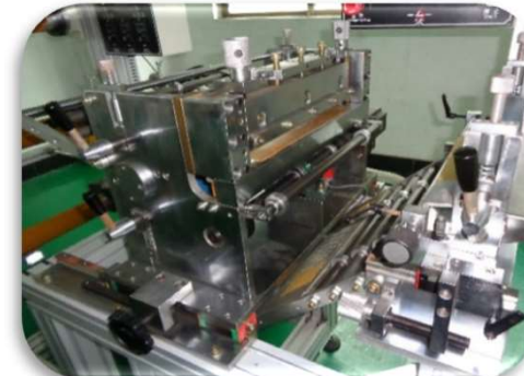
移載裁断機部
