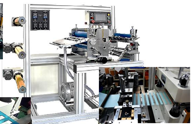
非同期移載カット連動供給機 Model LWY-350 適用材料幅：350 (mm)
